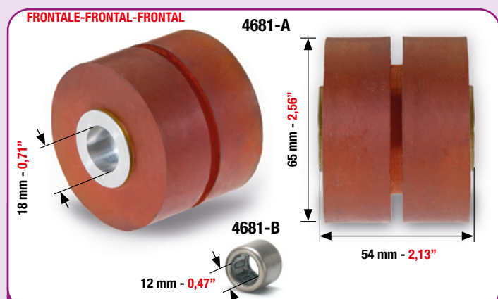
RUOTA DI TRASPORTO PER TAVOLA DI PUNTATURA (INTRODUZIONE) SHEET FEEDER WHEEL FOR ENTRY TABLE RUEDA DE TRANSPORTE PARA MESA DE REGISTRO (INTRODUCCION)
