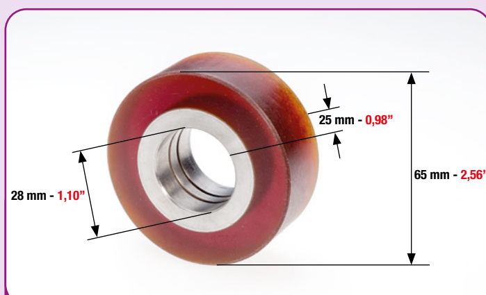
RUOTA DI INTRODUZIONE FOGLI PIANO DI PUNTATURA SHEET FEEDER WHEEL FOR ENTRY TABLE RUEDA DE INTRODUCCION DEL PLIEGO A LA MESA DE REGISTRO
